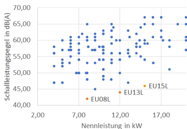
Marktvergleich Schallleistungspegel nach EN 12102
